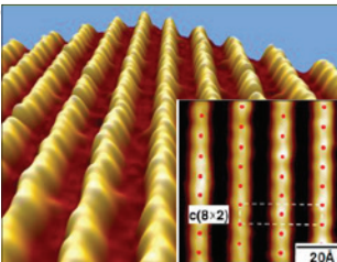
Anordnung von atomaren Goldketten auf einer Silizium(111)-Oberfläche
