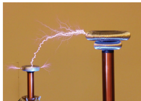
Hochspannungsexperimente mit Teslaspulen
