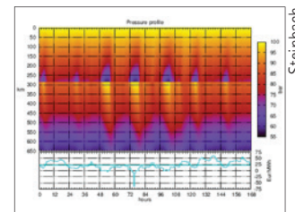
Optimaler Druckverlauf in einer Gaspipeline über eine Woche zum Ausgleich der Schwankungen regenerativ erzeugter elektrischer Energie mittels Druckreserve (»line pack«)
