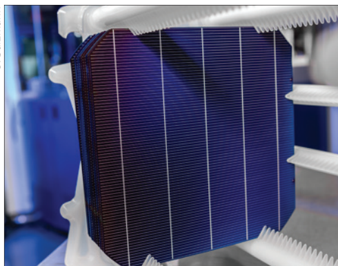
PERC-Solarzelle im 5-Busbar-Design mit 21,2% Wirkungsgrad. Dieser Wert war im April 2015 der Weltrekord für siebgedruckte Solarzellen.
