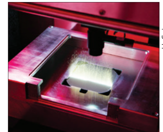
Am ISFH werden Laserprozesse zur Materialbearbeitung genutzt
