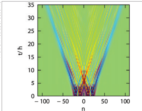
Simulation der Realzeitstreuung der Dynamik zweier Anregungen der Heisenberg Kette
