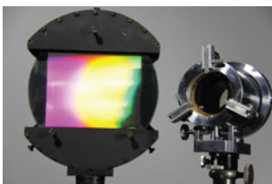
Wellenoptik mit Beugungsgitter
