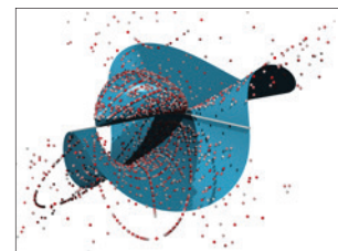
Rationale Punkte beschränkter Höhe auf einer singulären kubischen Fläche
