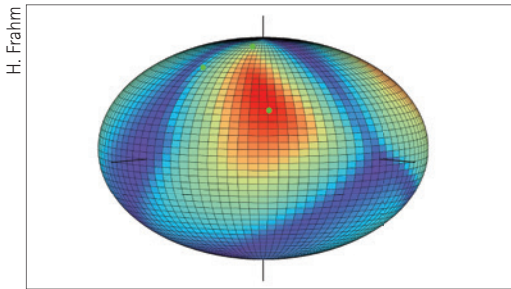
Phasendiagramm einer Kette von wechselwirkenden nicht-Abelschen Anyonen
