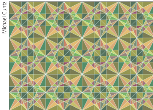
Ein affines kristallographisches Arrangement
