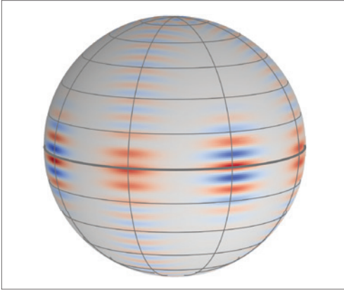
Wignerfunktion eines Spinzustandes eines Ensembles von verschränkten Uhrenatomen. Die Verschränkung der Atome kann die Stabilität einer Atomuhr verbessern.
