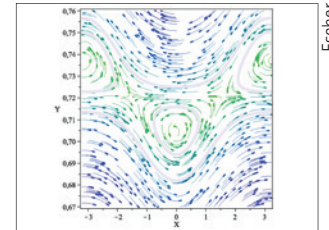
Stromlinien einer zweidimensionalen Strömung mit allgemeiner Wirbelverteilung
