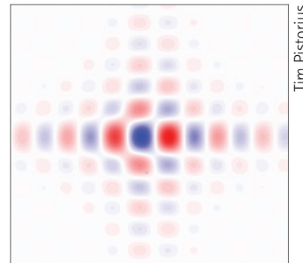
Quasiwahrscheinlichkeiten in einem offenen Quantensystem. Die blauen Bereiche zeigen nichtklassische Bereiche mit negativer Wahrscheinlichkeitsdichte an.
