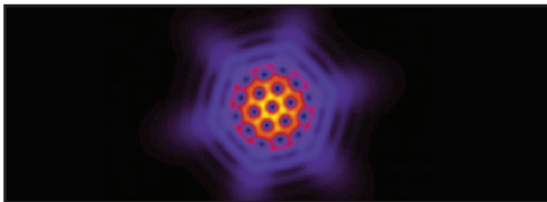
Gitterphase eines zweidimensionalen Bose-Einstein Kondensats mit synthetischer Spin-Bahn-Kopplung
