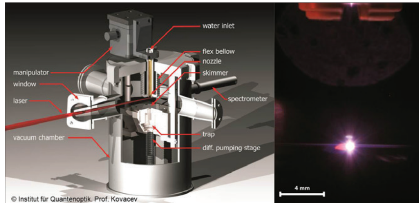
Experimenteller Aufbau zur Erzeugung von Harmonischen in Flüssigkeitsstrahlen. Der intensive Laserpuls erzeugt ein Plasma bei der Wechselwirkung mit einem Wassertropfen.
