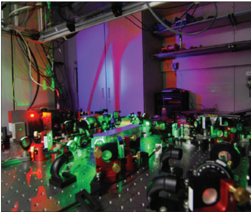
Optischer Tisch im Quantum Control Labor
