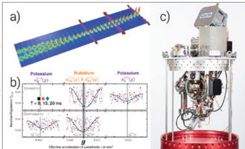
a) Interferenz eines Bose-Einstein-Kondensats; b) Signale eines Zwei-Spezies-Interferometers mit Rubidium und Kalium; c) Apparatur MAIUS-A für Höhenforschungsraketenmission
