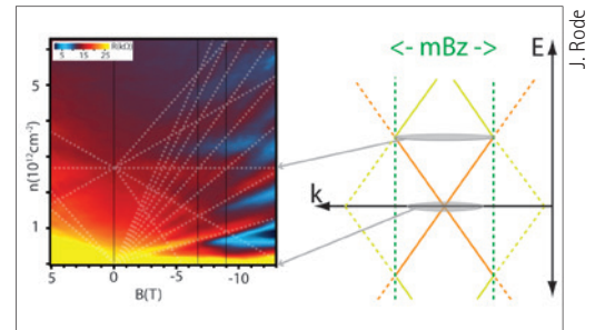
Beispiel einer Messung von Übergittereffekten in gefalteten Graphenstrukturen zusammen mit einem Schema der Bandstruktur
