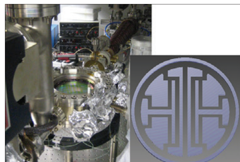
Links: UHV-Vakuumanlage zur Erzeugung ultrakalter NaK-Moleküle. Rechts: Elektrodenstruktur der Hauptkammer zur Kontrolle der molekularen Wechselwirkung durch E-Felder.
