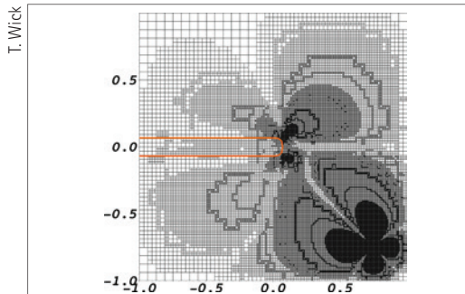
Adaptiv verfeinertes Gitter
