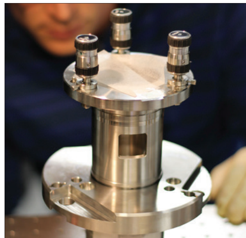
Zusammenbau eines hochauflösenden Objektivs zur Detektion einzelner Moleküle
