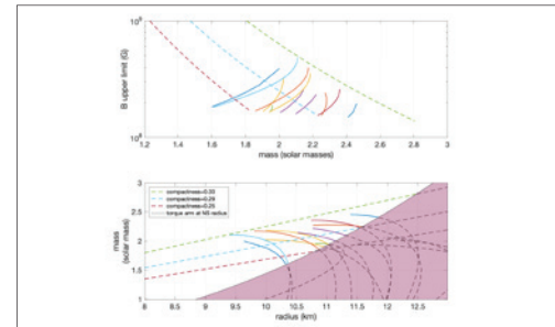
Scorpius X-1 Oberflächenmagnetfeldstärke und Masse-Radius Ausschlussregionen.
