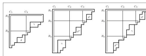
Tensorprodukte: Reduktionen an Young-Tableaux
