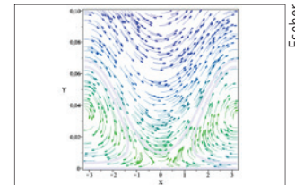
Stromlinien einer zweidimensionalen Strömung mit allgemeiner Wirbelverteilung
