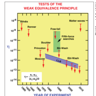
Seit den ersten Präzisionsexperimenten des Ungarn Baron Lorand Eötvös in den Jahren 1906-09 wurde die Gleichheit der schweren und trägen Masse mit einer um fünf Größenordnungen gesteigerten Genauigkeit überprüft. Die MICROSCOPE Mission fügt weitere zwei Größenordnungen hinzu.
