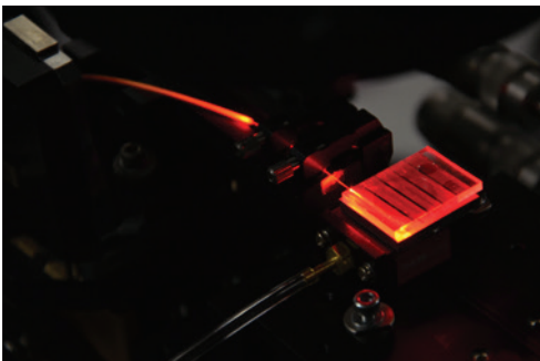
Faseroptische Messkonfiguration zur Validierung integriert-optischer Foliensensoren, die mittels additiver Fertigung realisiert werden
