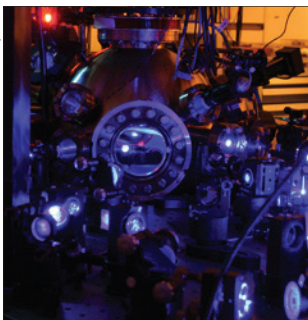
Bildunterschrift: Strontium-Atomwolke bei wenigen Millikelvin über dem absoluten Nullpunkt in der optischen Gitteruhr der PTB
