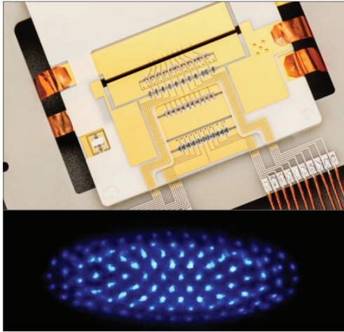
Oben: Präzisions-Ionenfalle aus AlN-Keramik mit insgesamt acht Fallen-Segmentierungen, Unten: Lasergekühlter Ionen-Coulomb-Kristall aus Ytterbium-Ionen, der in einem der Fallensegmente gespeichert ist.
